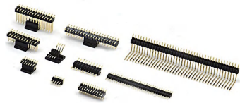
1.00mm 排针 PH1007系列
