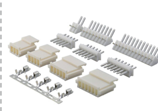
2.50mm 线对板 A2504系列
