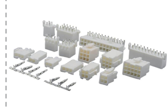
4.14mm 线对线 C4140系列
