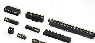
1.00mm 排母 FH1007系列
