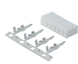
2.00mm 板对板 B2001系列
