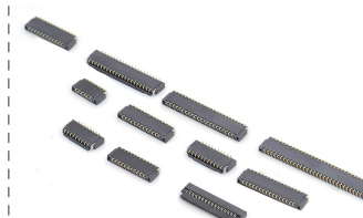
0.30mm FPC FFC F0303系列
