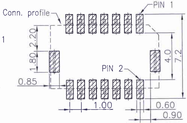
P.C.B. LAYOUT
