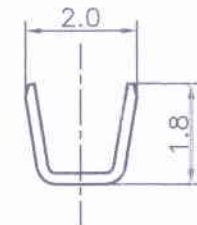
Section D-D
