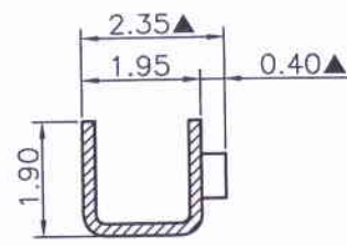
SECTION D-D
