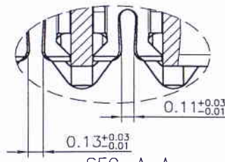
SEC: A-A SCALE: 2.5:1
