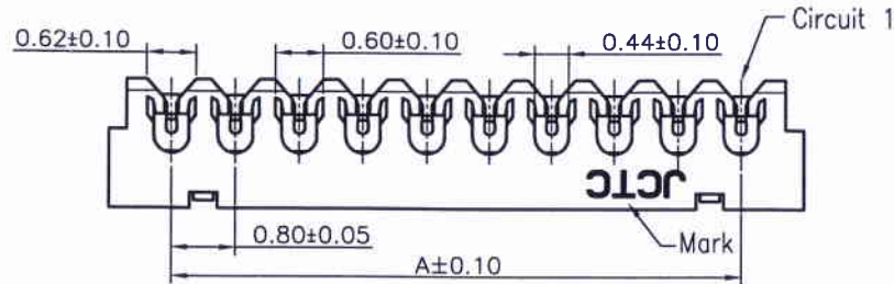
DETAIL "A" SCALE: 2:1
