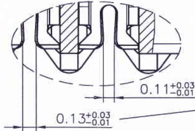
SEC: A-A SCALE: 2.5:1
