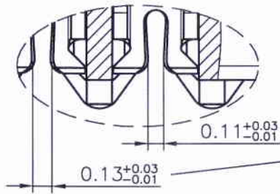
SEC: A-A SCALE: 2.5:1
