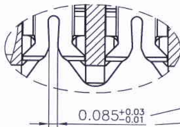
SEC: A-A SCALE: 2.5:1
