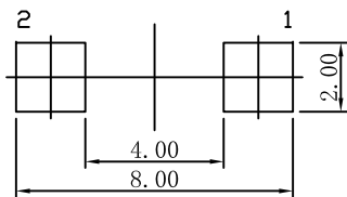
印刷板安装孔图 P.C.B Mounting pattern dimension
