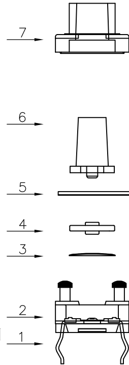
产品零部件剖析图
