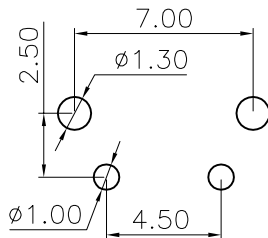
印刷电路板开孔
