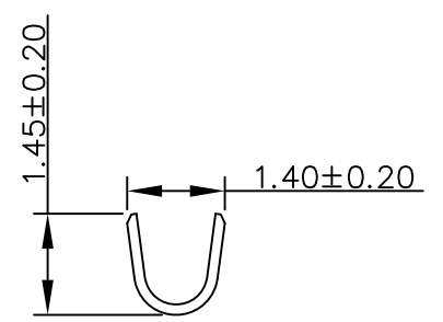
剖视图:B-B
